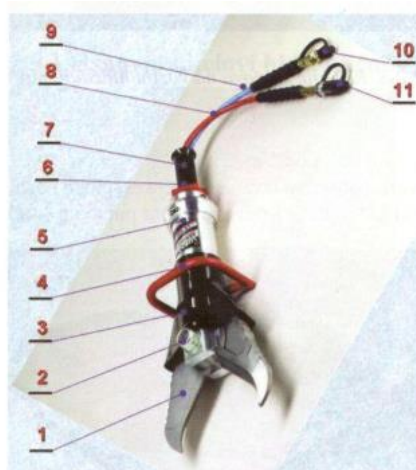
Slika 9. Hidraulične škare [1]
