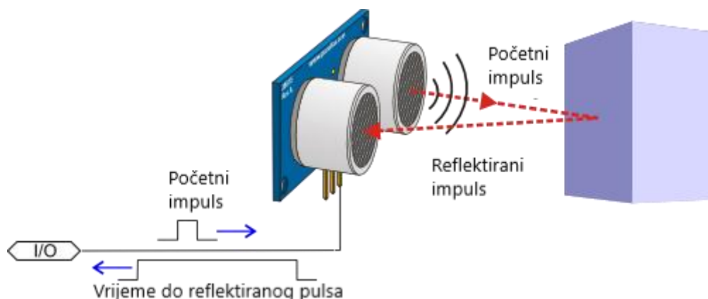
Slika 5. Predodžba načina rada ultrazvučnog senzora.[2]
