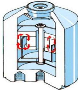
Slika 15. Predodžba kontaktnog senzora brzine.[8]
