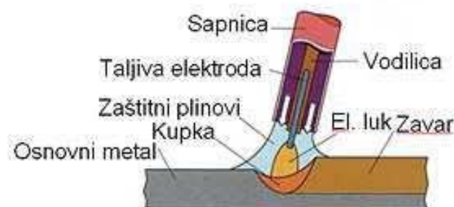
Slika 24. MIG/MAG zavarivanje
