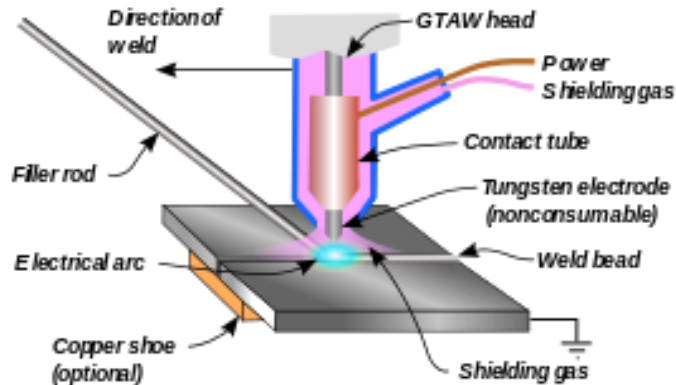
Slika 25. TIG zavarivanje
