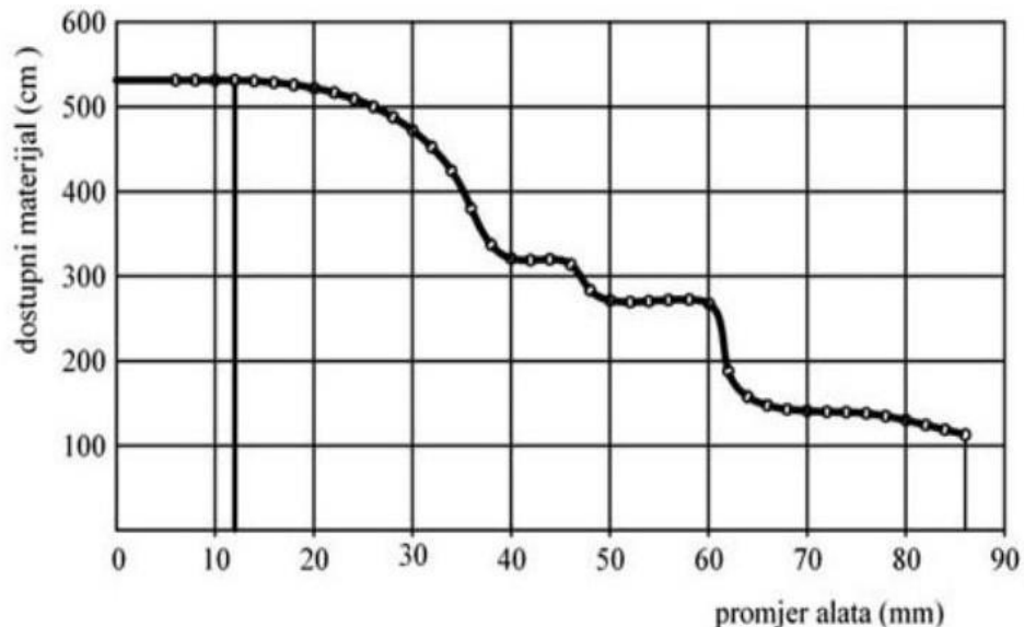
Slika 12: TAD krivulja
