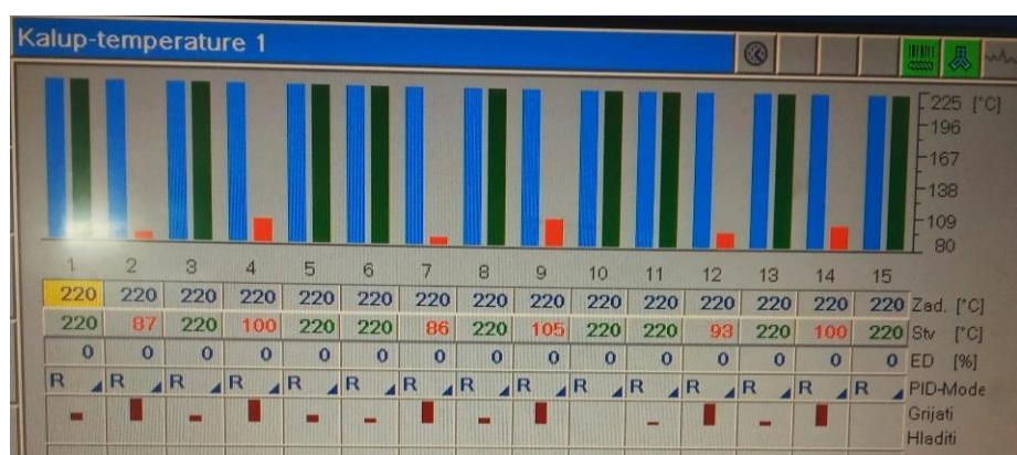
Slika 36. Temperature kalupa prilikom optimiranja
