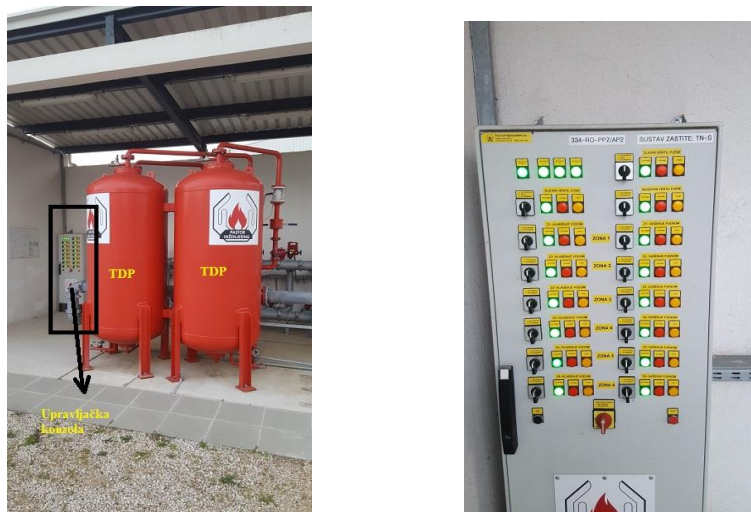
Sl. 13. Poluautomatska aktivacija drencher sustava
