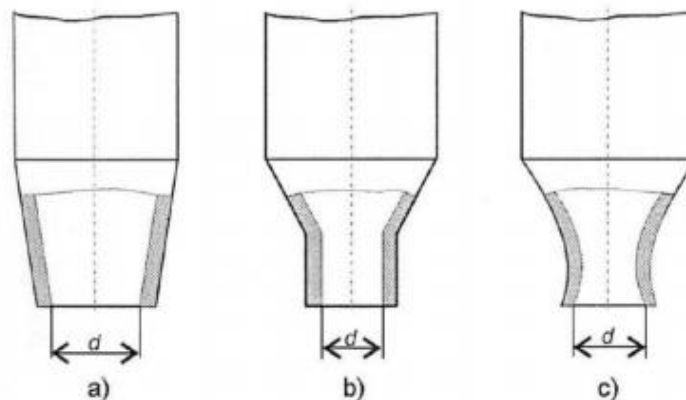
Slika 6. Najčešće korištene izvedbe sapnica [10]
