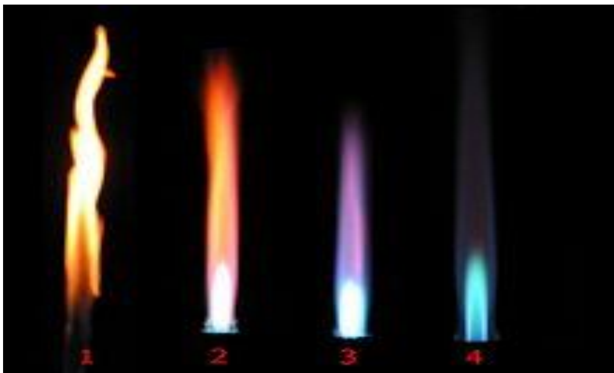
Slika 6. Različite vrste plamena kod Bunsenovog plamenika.[6]
