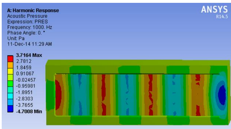
Slika 20. Konture zvučnog tlaka.[15]
