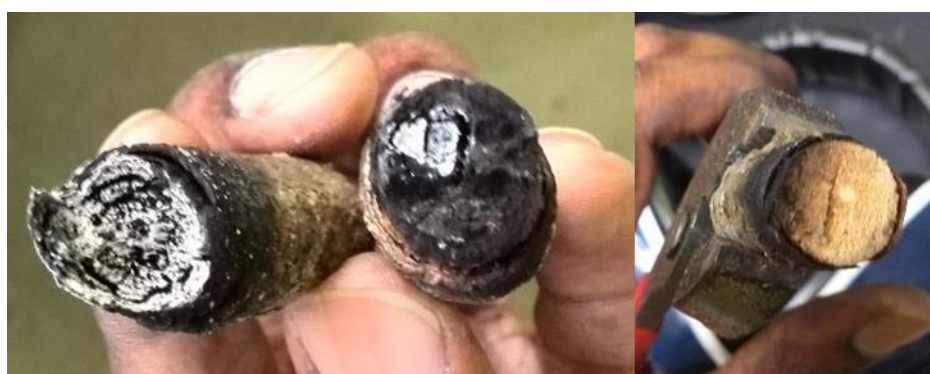
Slika 27. Penetracija vatre u drvetu.[15]
