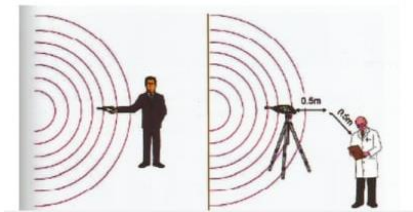
Slika 6. 4. Položaj operatera
