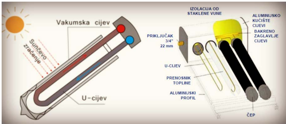
Slika 4. Toplinska cijev [2]
