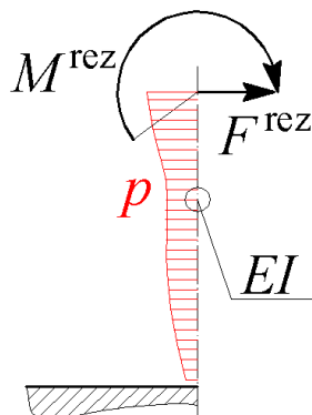
Slika 29. Predodžba proračunskog modela deformiranja spremnika. Izvorno autor.
