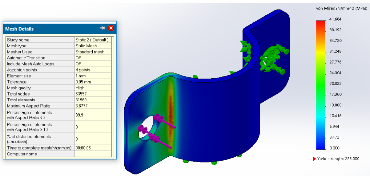
Slika 53. Prikaz simulirane obujmice i rezultata napreznja
