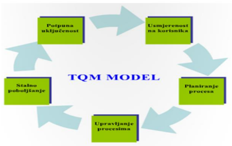
Slika 2. Model TQM-a
