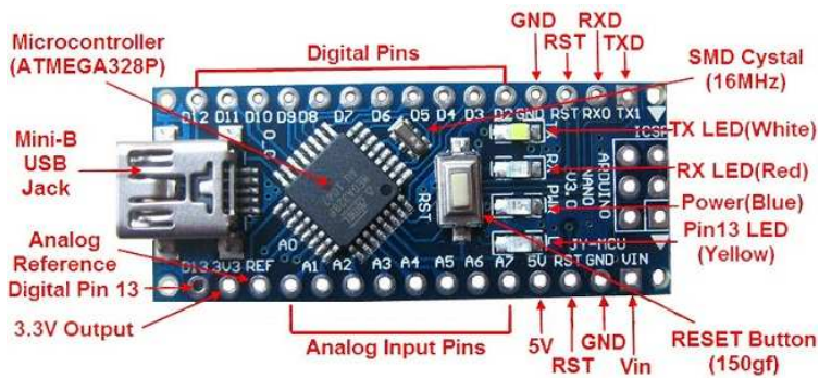
Slika 23: Arduino Nano [18]
