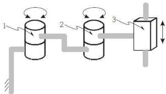
Slika 7: SCARA konfiguracija [3]
