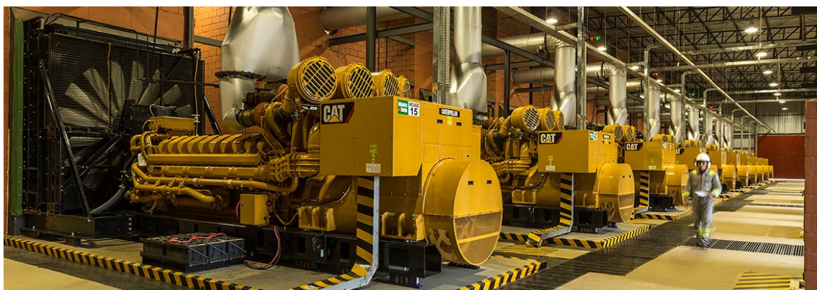
Slika 15. Izgled paralelno spojenih generatora u potpalublju platforme
