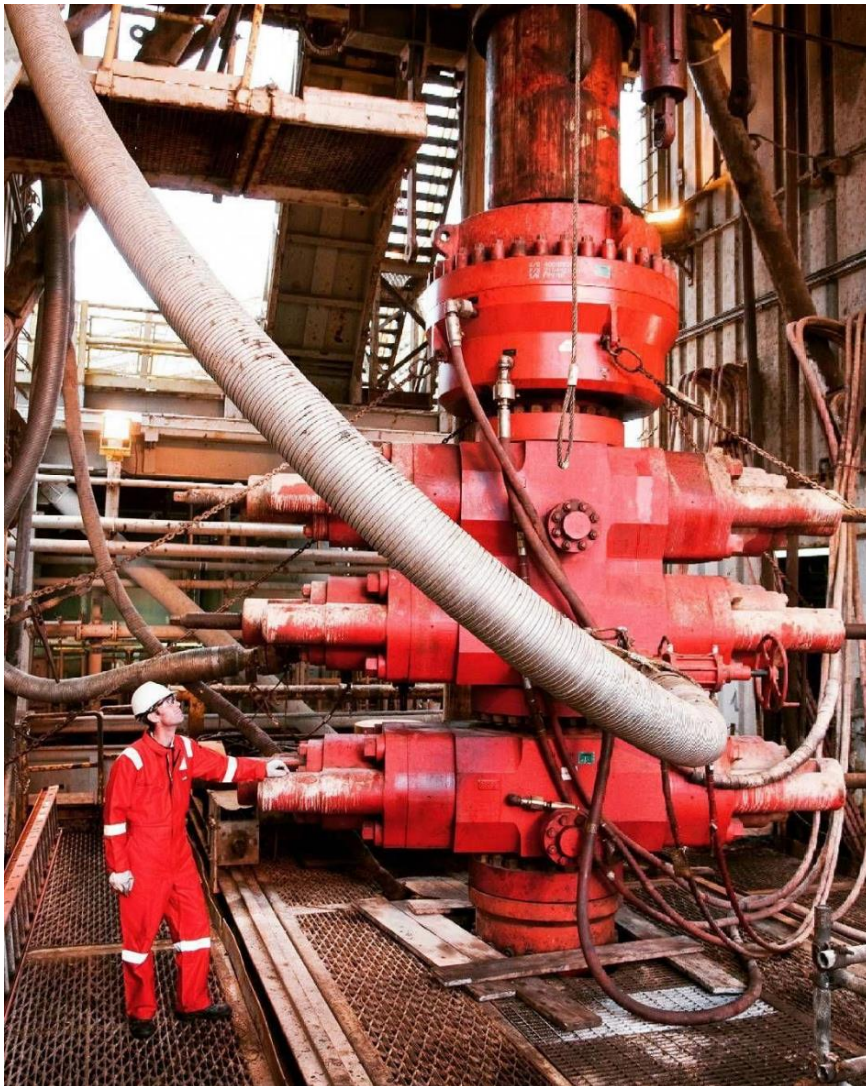
Slika 25. Prikaz BOP uređaja na kopnoj bušačkoj garnituri
