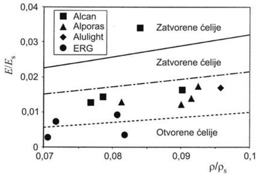
Slika 24. Ovisnost relativnog modula elastičnosti o relativnoj gustoći [1]
