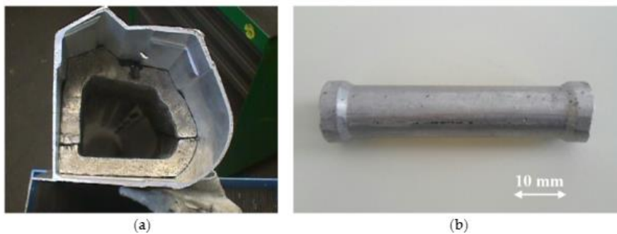
Slika 46. a) Al pjenasti dio za Ferrari 360 b) mali element koji apsorbira pad sustava za Audi Q7 [12]
