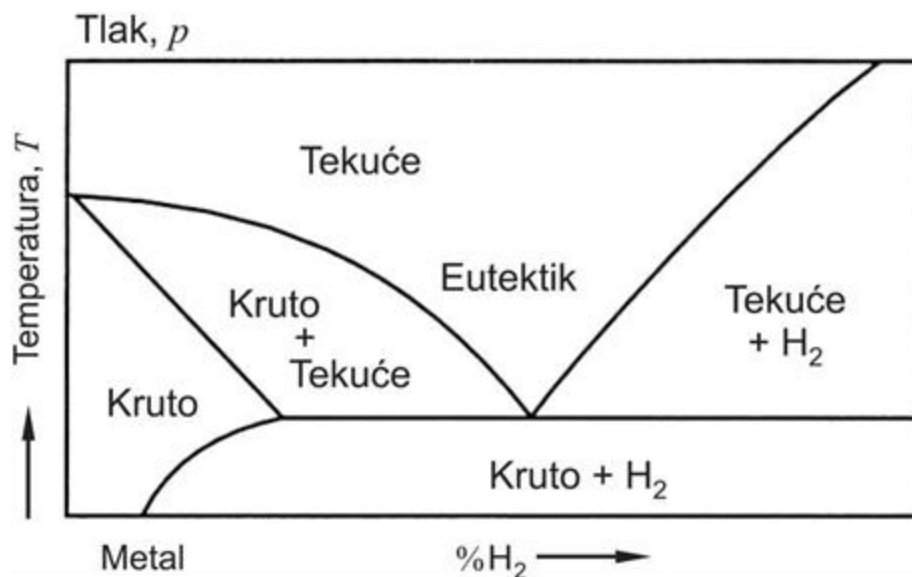
Slika 16. Binarni dijagram stanja metal-vodik [1]
