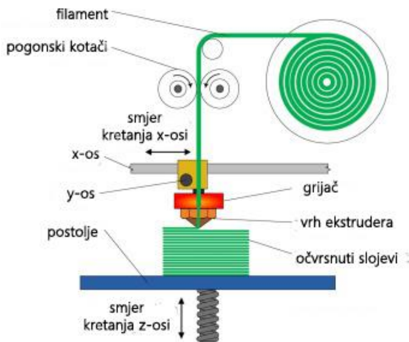
Slika 17. FDM tehnologija [17]
