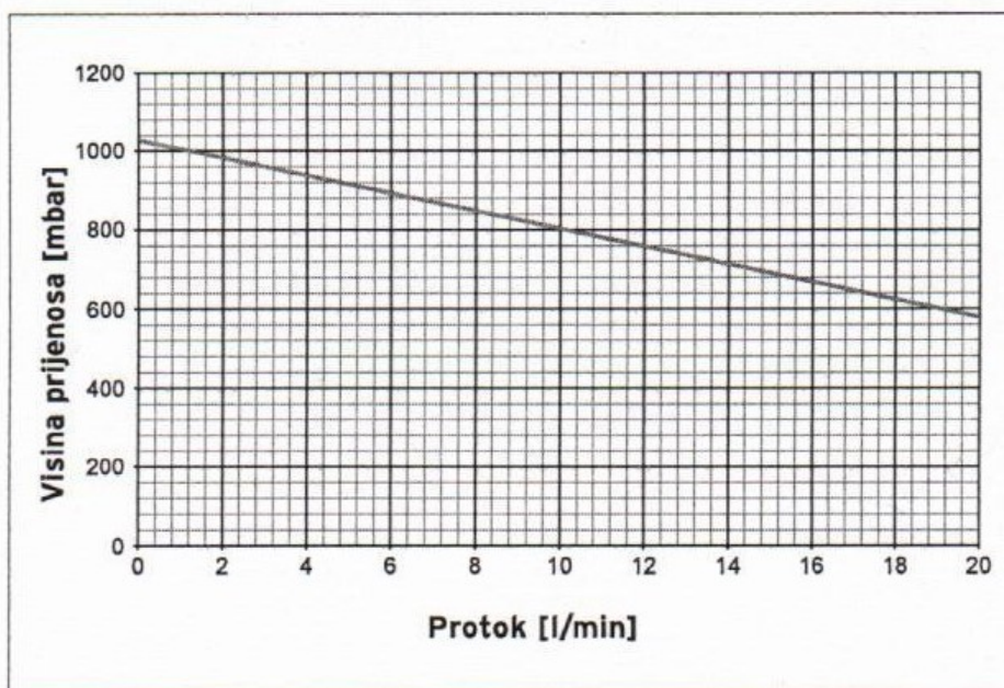
Slika 33. Visina dobave solarne crpke – VMS 70
