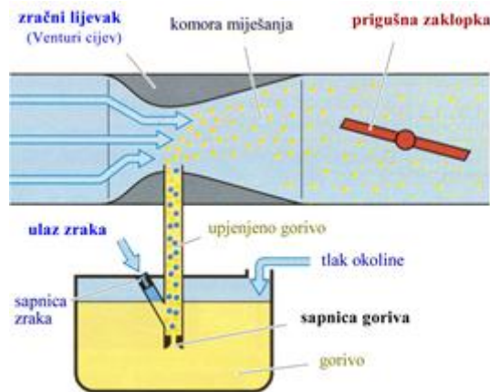
Slika 21. Princip rada karburatora
