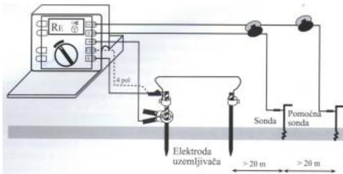
Slika 26. Predodžba mjerenje otpora uzemljenja pomoću strujnih kliješta i sonde [14]
