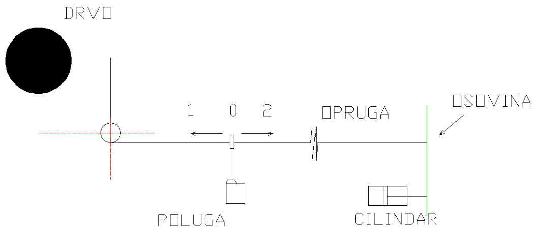
Slika 35. Regulacijska shema
