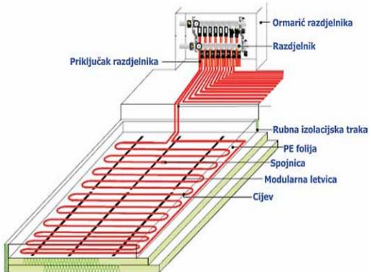
Slika 5.5. Elementi sustava podnog hlađenja [14]
