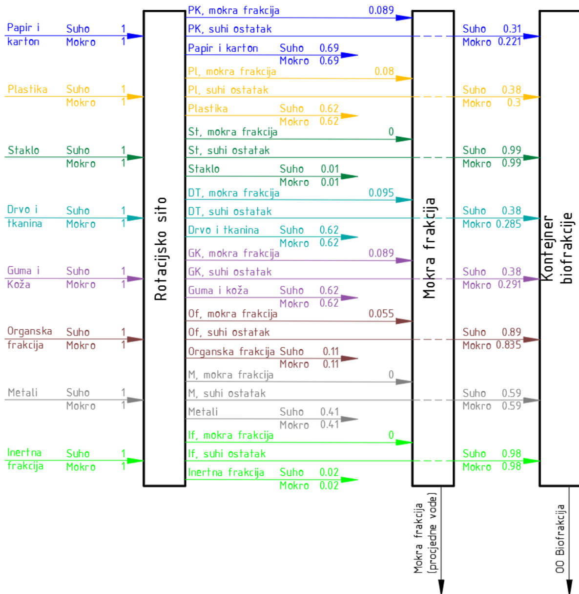
Slika 18. Shema rotacijskog sita s transfer koeficijentima masenih tokova
