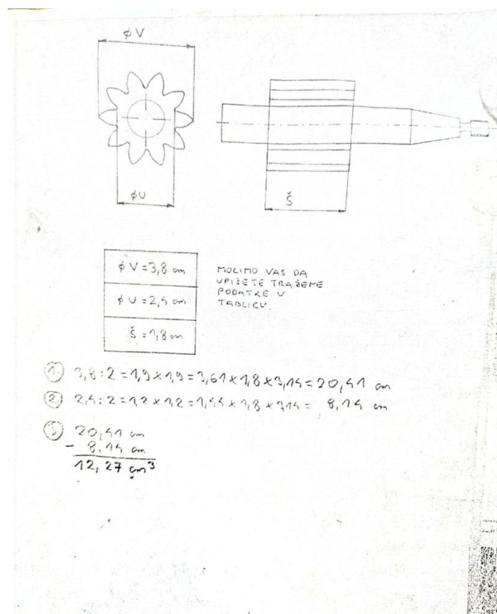
Slika 53. Zupčanici zupčaste pumpe
