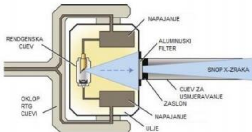
Slika 14. Rendgenska cijev
