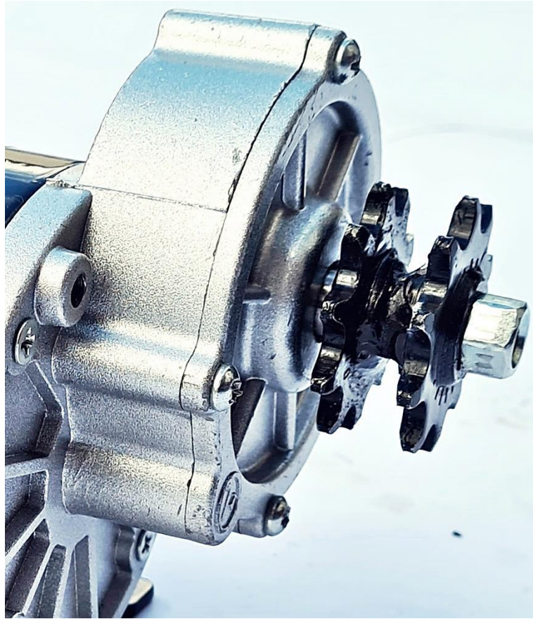
Slika 44 – Prikaz duplog lančanika montiranog na osovini elektromotora.
