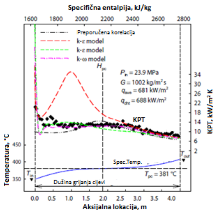
Slika 2-20: Usporedba vrijednosti koeficijenta prijelaza topline i temperature stijenke cijevi izraĉunatih korelacijom (2) i CFD-raĉunalnim paketom FLUENT [28] s eksperimentalnim podacima duĉ 4 m duge kruĉne cijevi promjera D=10 \text{ mm} : P_{in} = 23,9 \text{ MPa} i G=1002 \text{ kg/m}^2
