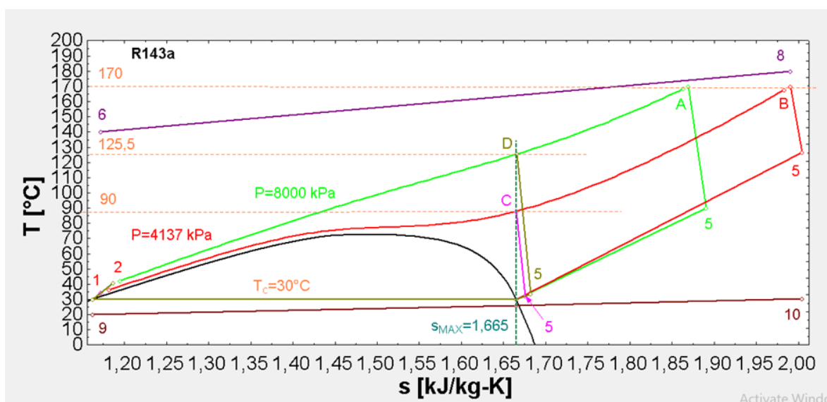
Slika 4-91: Prikaz danog ORC ciklusa s karakterističnim točkama (A, B, C i D) nadkričnog radnog područja za radni fluid R143a
