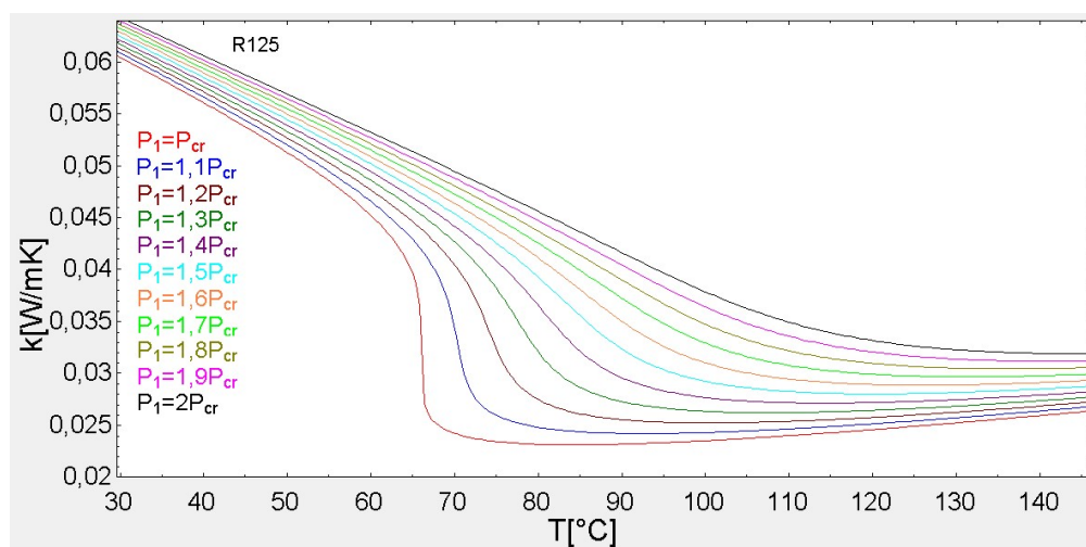
Slika 4-30: Prikaz promjene vrijednosti koeficijenta toplinske vodljivosti o temperaturi uslijed povećanja vrijednosti nadkričnog tlaka za radni fluid R125
