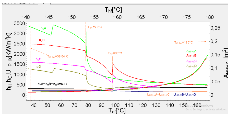
Slika 4-84: Prikaz promjene vrijednosti koeficijenta prijelaza topline ( h_H, h_C ), ukupnih koeficijenta prolaza topline ( U_{HPHX} ) i površina segmenata izmjenjivača topline ( A_{HPHX} ) duž razmatranog izmjenjivača topline za radni fluid R32
