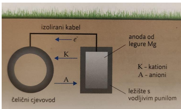
Slika 15. Protektorska zaštita [1]
