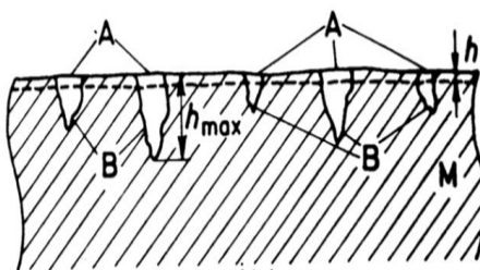
Slika 6: Jamičasta korozija, A-površina metala prije korozije, B-površina metala nakon korozije, M-materijal, h-prosječna dubina prodiranja korozije, h max -maksimalna dubina prodiranja korozije [7]
