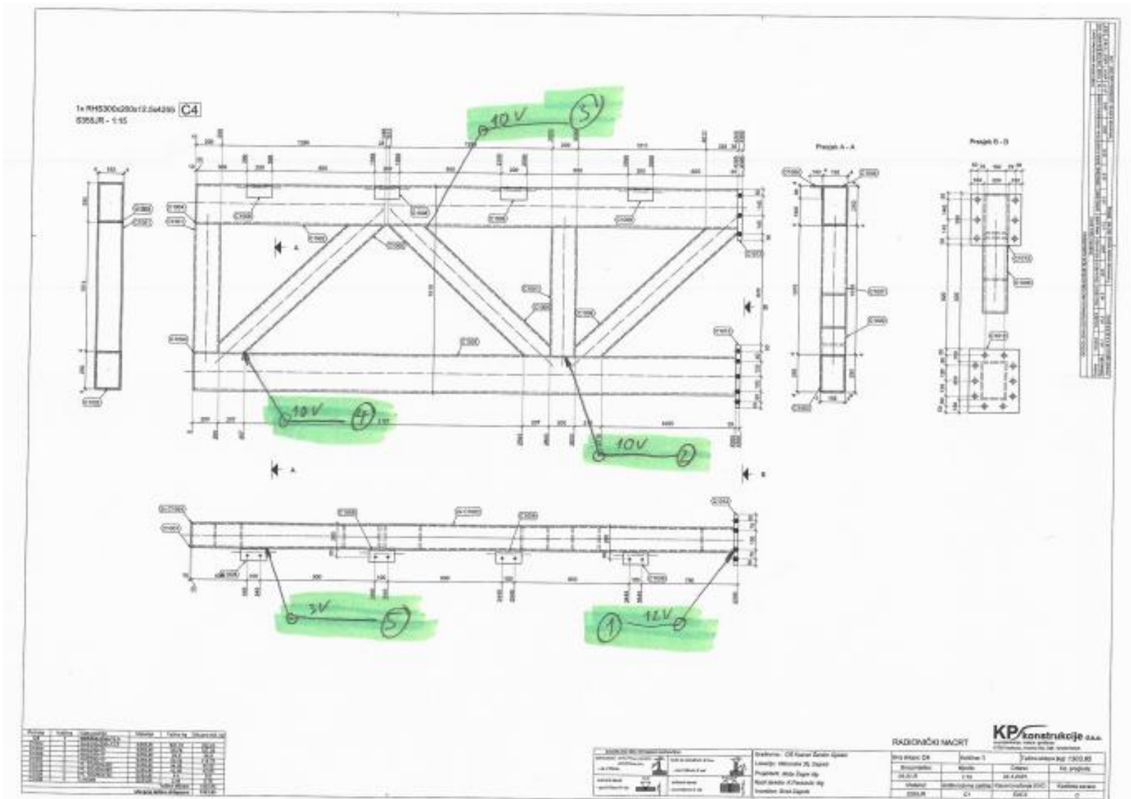
Slika 29. Sklop C4
