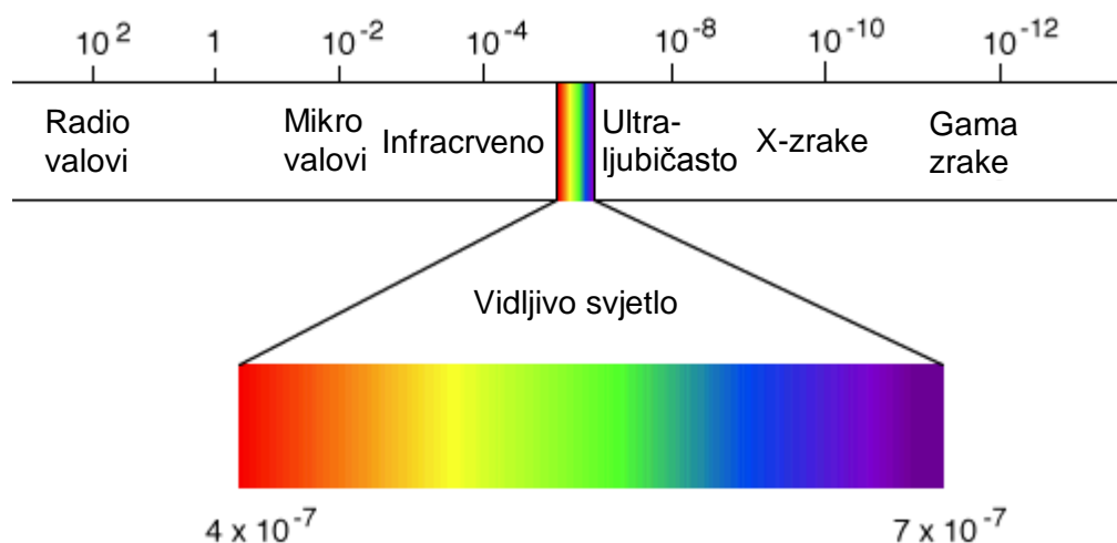
Slika 15. Elektromagnetski spektar [ 12 ]
