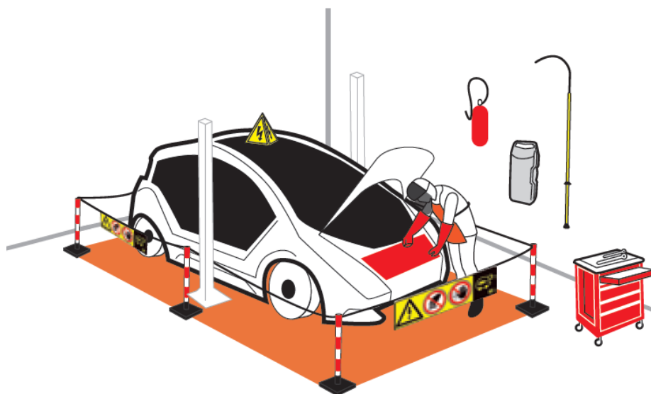
Slika 19. Zona opasnosti [17]
