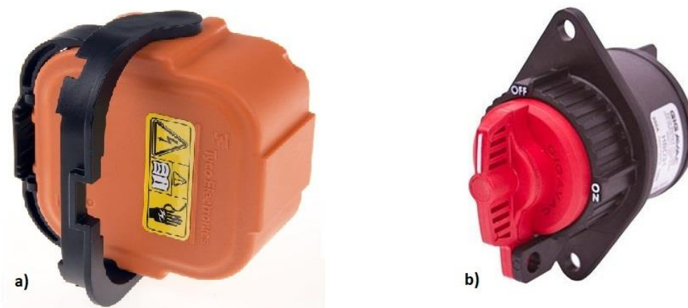
Slika 23. Servisni prekid: a) konektor [28], b) sklopka sa mogućnošću zaključavanja u isključenom položaju [29]
