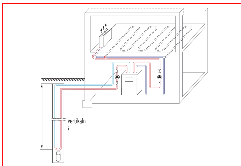
Slika 4.11. Kvalitativan prikaz dizalice topline tlo-voda, vertikalna izvedba izmjenjivača u tlu [17]
