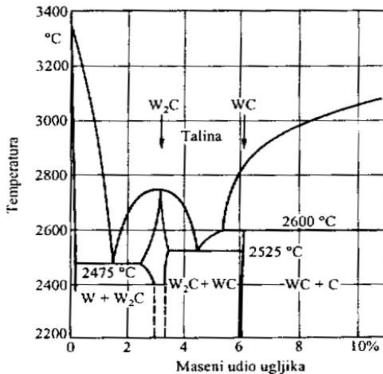
Slika 3. Fazni dijagram W-C sustava [2]
