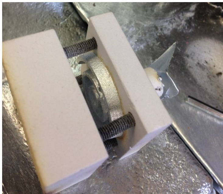
Slika 29. Otvoravanje Kalupa 1 nakon skrućivanja litine
