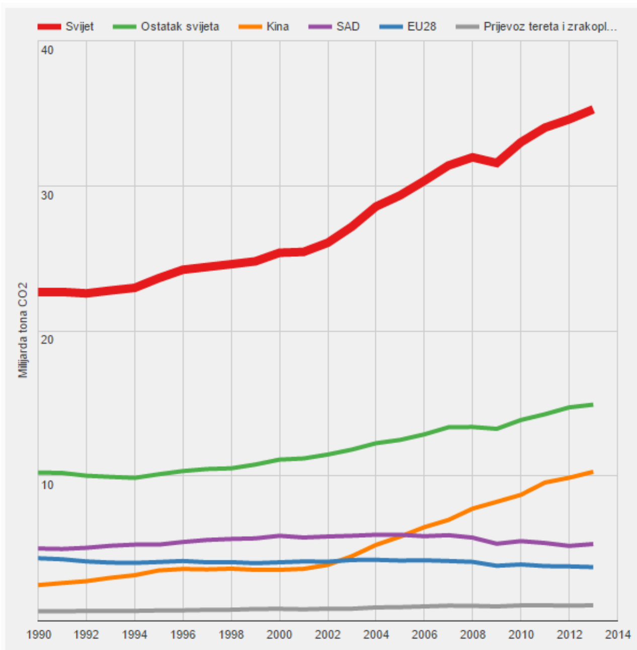
Slika 7.1. Svjetski udio u emisijama CO 2
