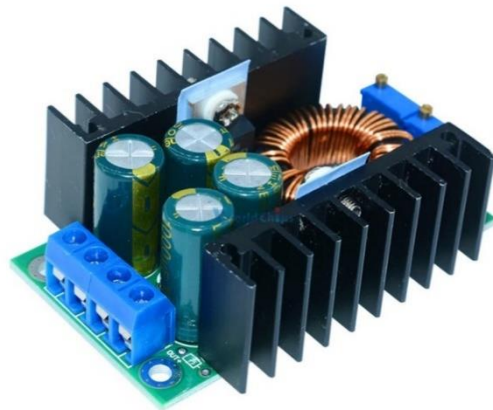
Slika 40. Izgled DC-DC silaznog prekidačkog naponskog regulatora [49]
