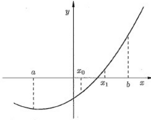
Slika 6. Raspolavljanje intervala [a, b]
