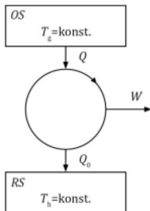
Slika 19. Shema toplinske pumpe [4]
