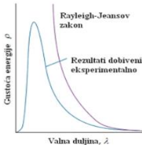
Slika 2. Graf razlike između eksperimentalnih rezultata i krivulje dobivene Rayleigh Jeansovim zakonom [13]
