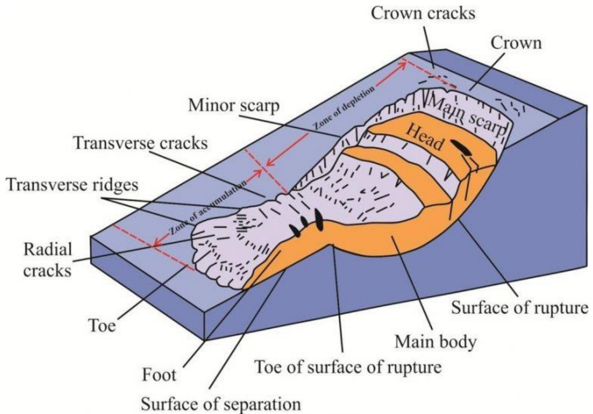
Slika 6. Elementi klizišta.[8]
