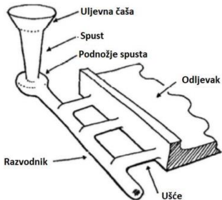
Slika 16. Uljevni sustav [12]
