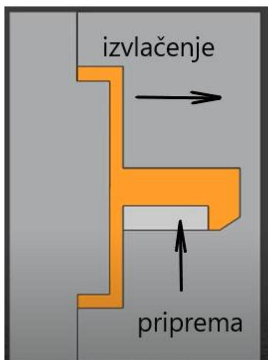
Slika 8. Izbjegavanje podrezivanja [5]
