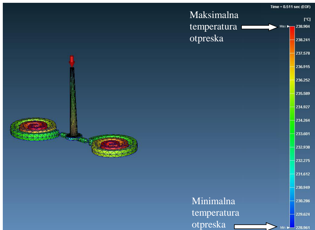
Slika 71. Raspon temperatura otpreska na kraju procesa
