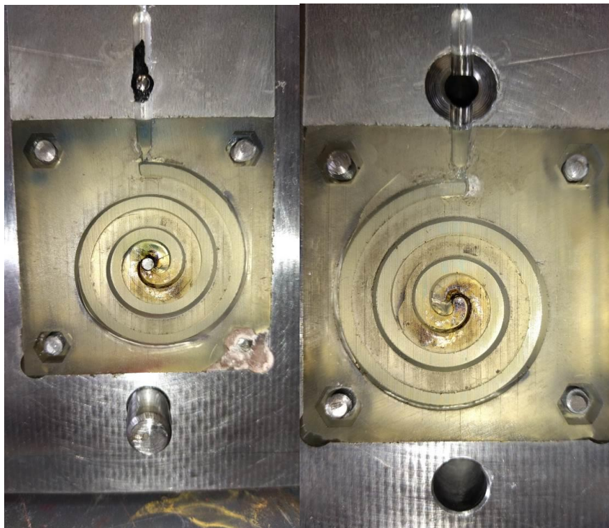
Slika 67. Izgled polimernog kalupa nakon šezdeset otpresaka
