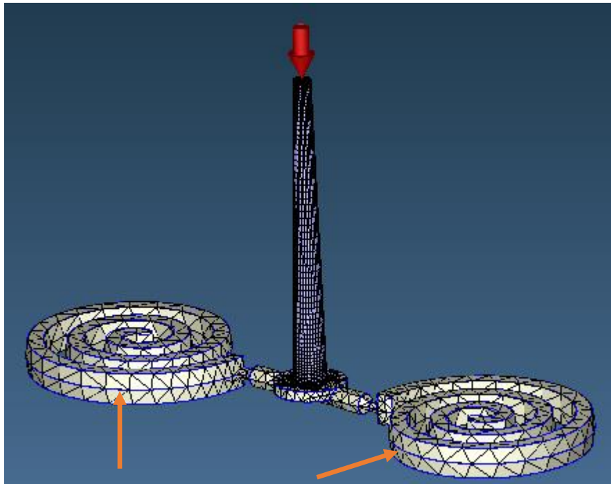
Slika 73. Linija spajanja
