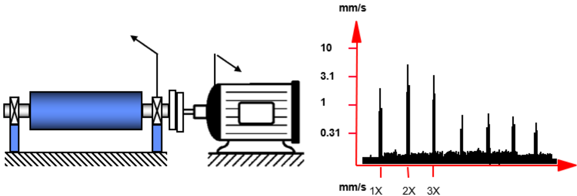
Slika 37. Shema paralelne necentričnosti sa pripadajućim frekvencijskim spektrom ; Izvorno autor
