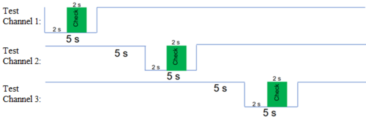
Slika 56. Grafički prikaz testiranja kanala ; Izvorno autor
