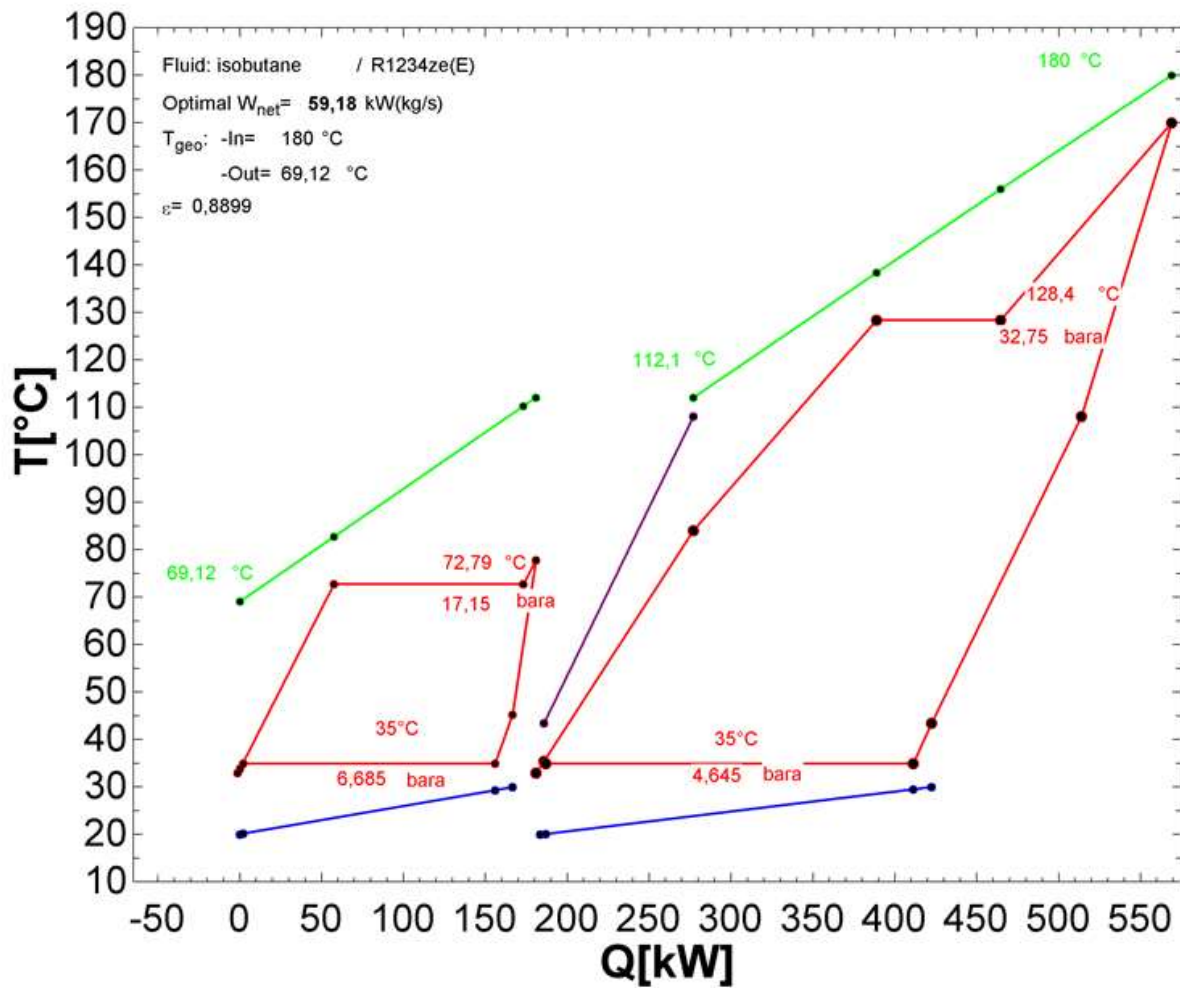
slika 38. T-Q dijagram Isobutane/R1234ze(E)
