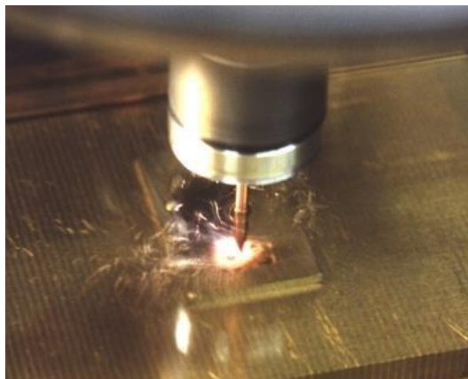
Slika 4 Proces elektroerozije [4]
