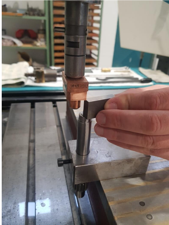
Slika 59 Uzimanje visine erodiranja pomoću etalona
