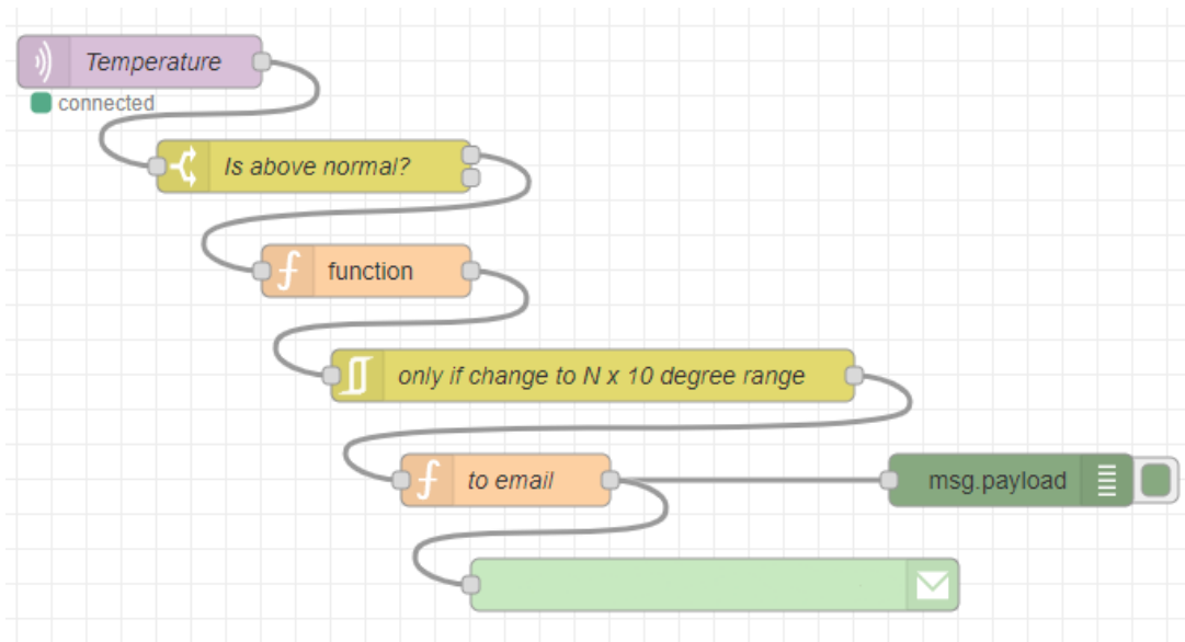
Slika 18. NodeRed kompozicija
