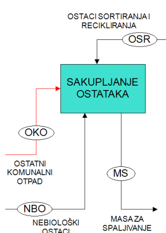
Slika 114. Blok shema sekcije za sakupljanje ostataka.
