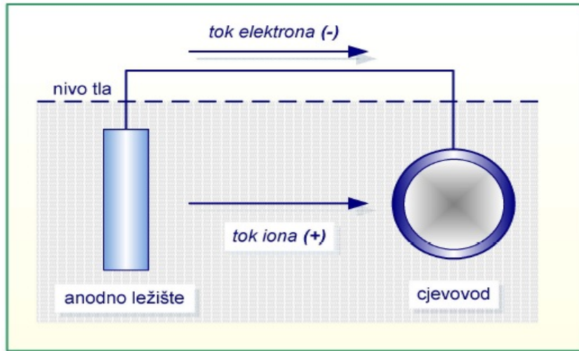
Slika 6. Shema sustava katode zaštite sa žrtvenim anodama
