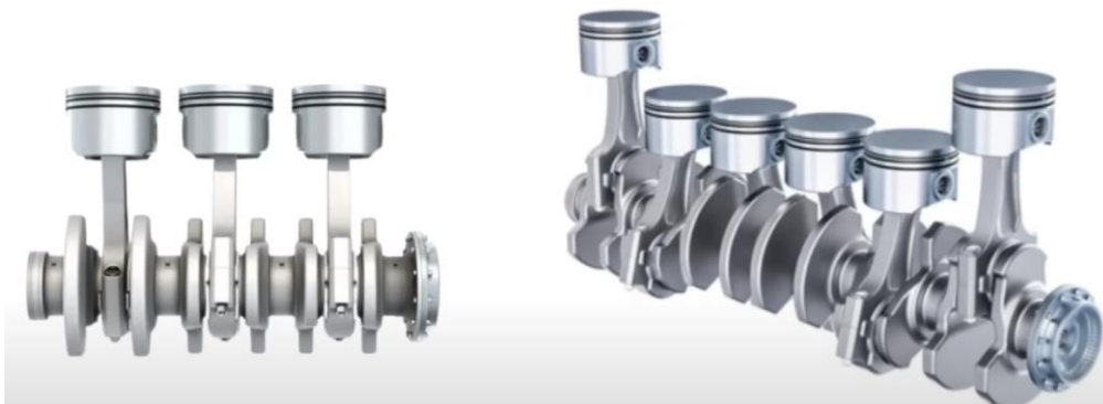
Slika 47. Raspored klipova u trocilindričnom i šesterocilindarskom motoru [8]
