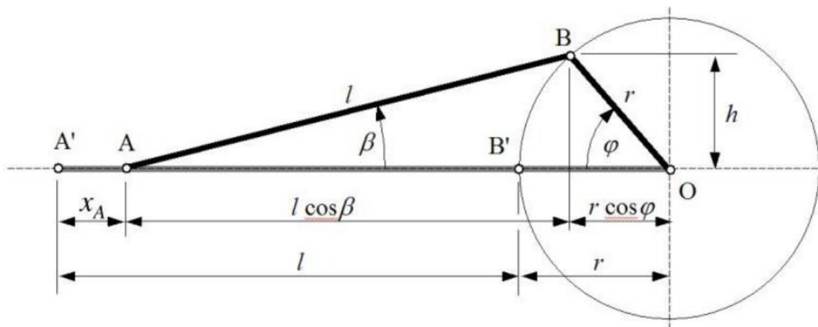
Slika 14. Hod klipa [3]
